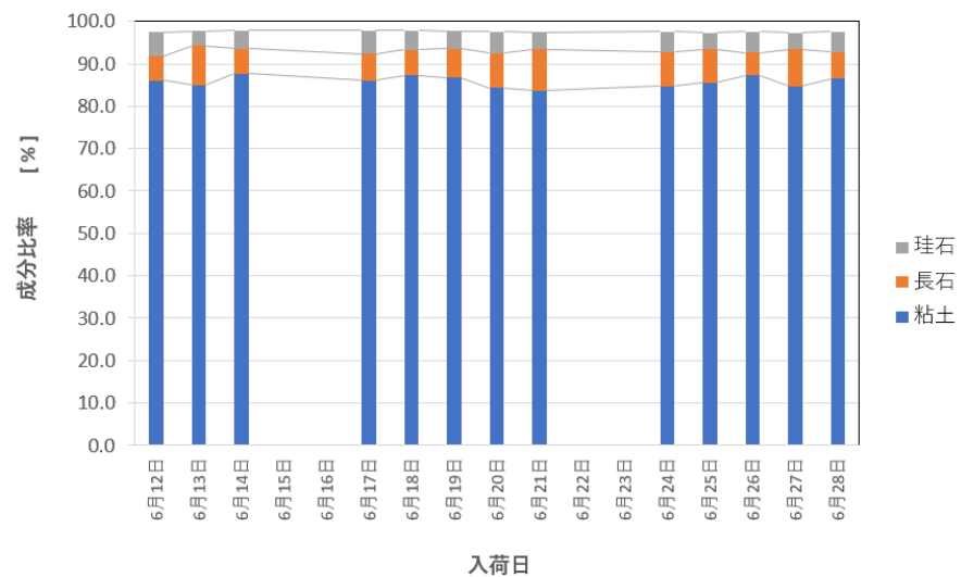
水簸後の蛙目粘土 成分変動
