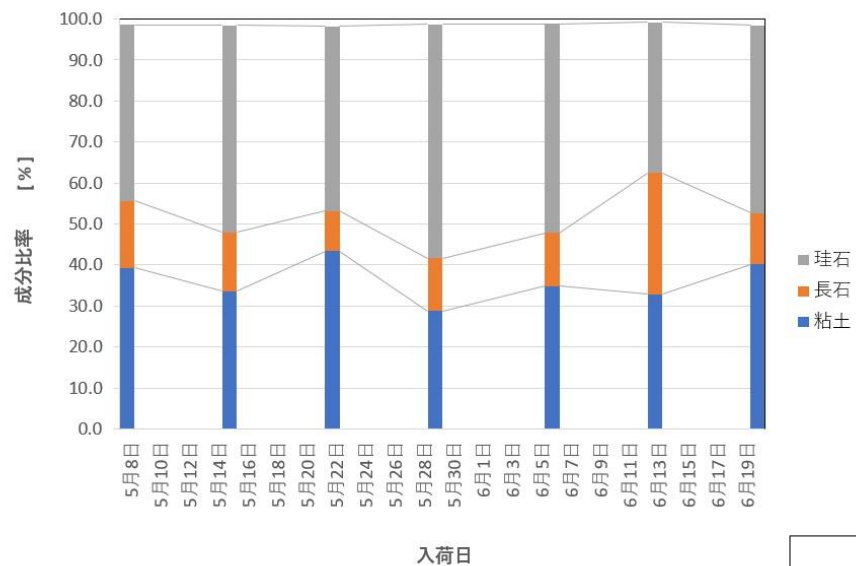
蛙目粘土の原土の成分変動
