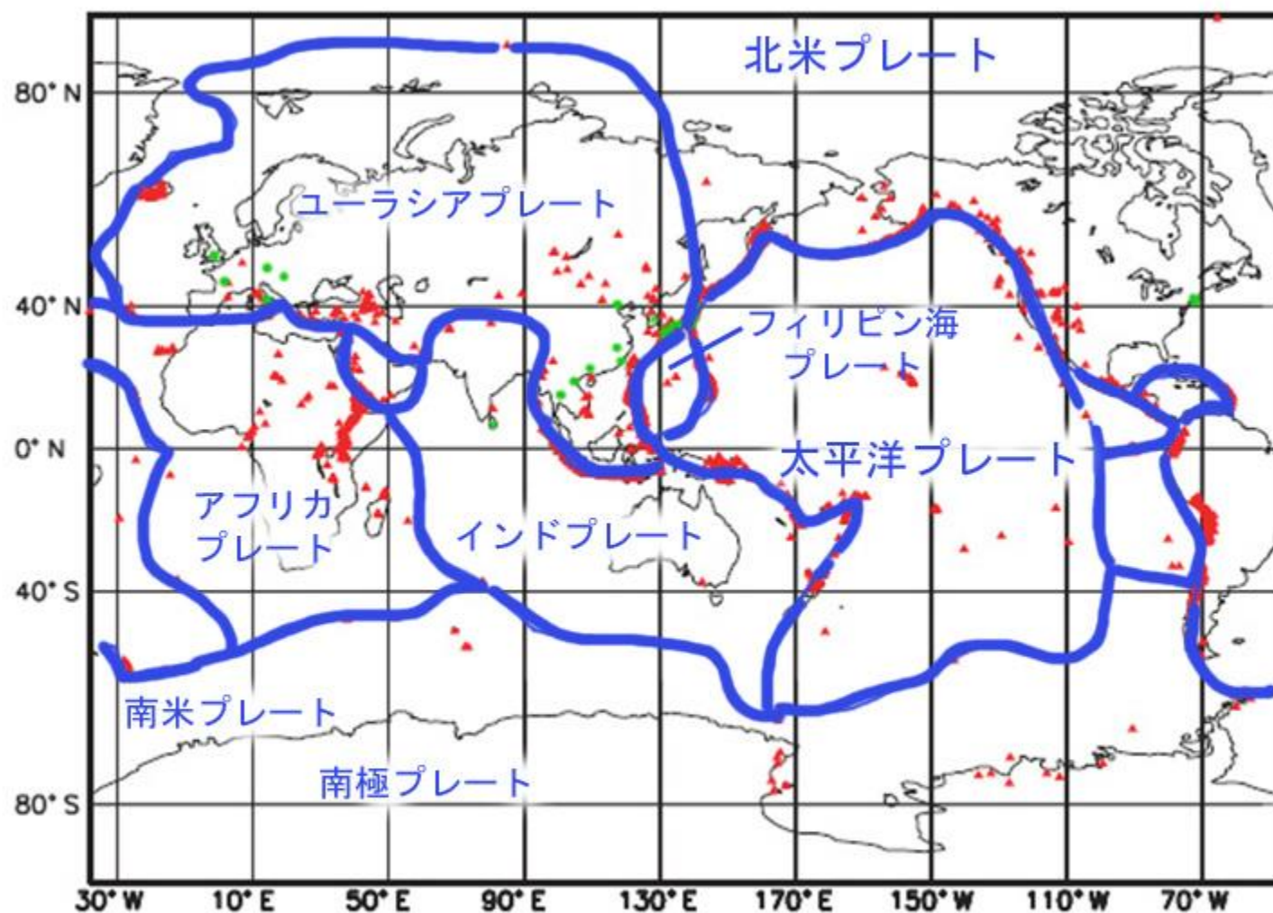
図 1-1-3 世界の主な火山 主な窯業地
